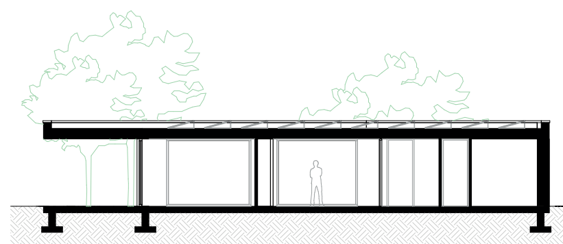
langsdoorsnede
